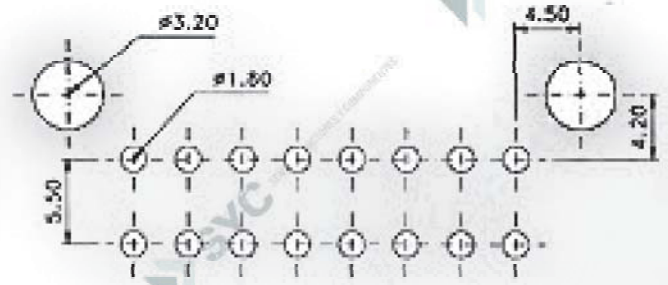
P.C.B. LAYOUT
