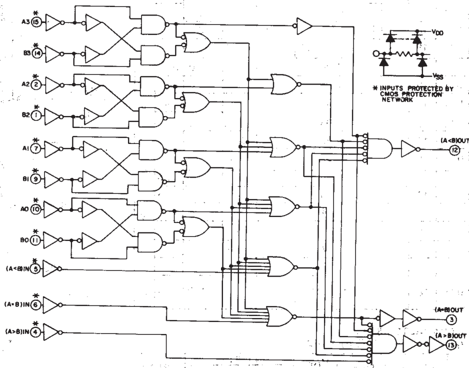
Fig. 4 - Logic diagram.
