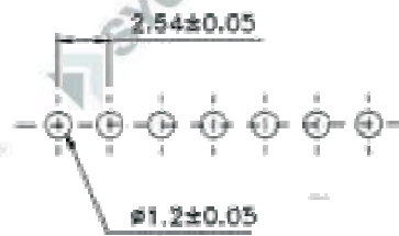
P.C.B. LAYOUT
