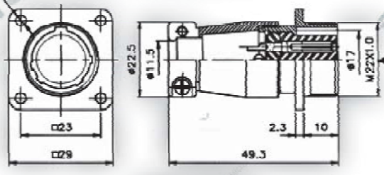
PLS-20-AD(F)
