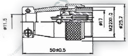
PLS-20-ADF
