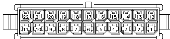
22PIN
