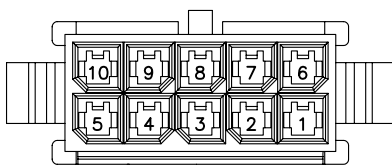
10PIN
