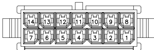
14PIN
